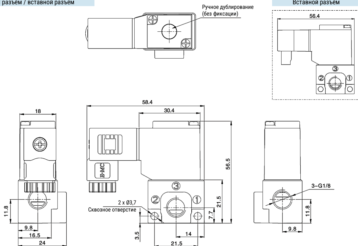
Индивидуальный распределитель ЕНЕ35А DIN разъем / вставной разъем
