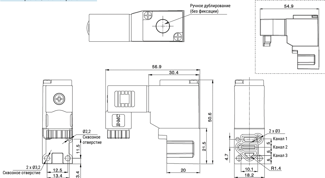
Стыковой распределитель ENE35M DIN разъём / вставной разъём
